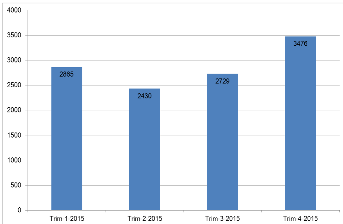
Figura nr.3: Numărul donatorilor de CSH recrutați și înscrși în RNDVCSH, pe trimestre, anul 2015
